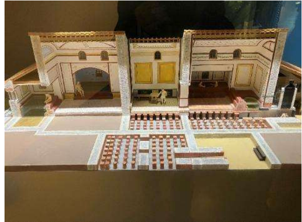
Die Therme im Schnittmodell mit aufgedeckter Fußbodenheizung.
